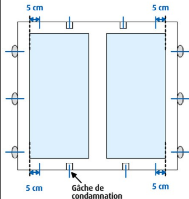
Illustration 25 : Disposition des fixations principales pour les fenêtres à ouverture à la française avec système de fermeture à renvoi d'angle en face 1 à 4 d'une construction dans la zone 20-50 mbar
