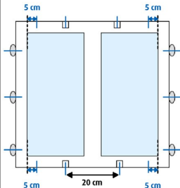
Illustration 24 : Disposition des fixations principales pour les fenêtres à ouverture à la française à deux vantaux munies d'un système de fermeture à sortie de tringle en face 1 à 4 d'une construction dans la zone 20-50 mbar
